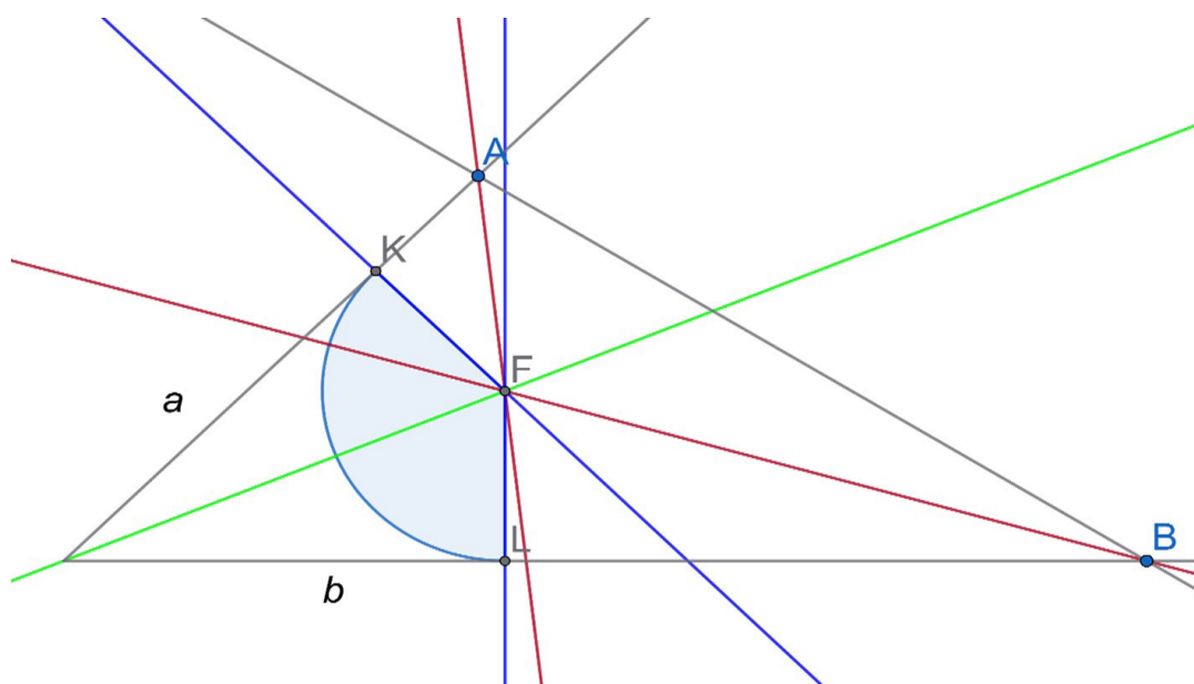
Рисунок 1: Построение биссектрисы угла с недоступной вершиной методом геометрической симметрии
