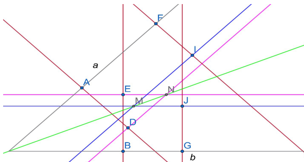
Рисунок 1: Построение биссектрисы угла с недоступной вершиной методом равных расстояний
